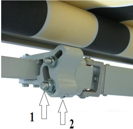
1 = Klemmschraube 2 = Stellschraube
